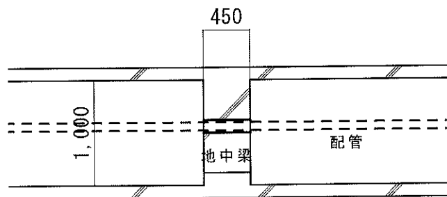
廊下床下に設ける通常のピット
